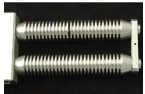
Ölkühler zum separaten Anbau. Material Aluminium.
